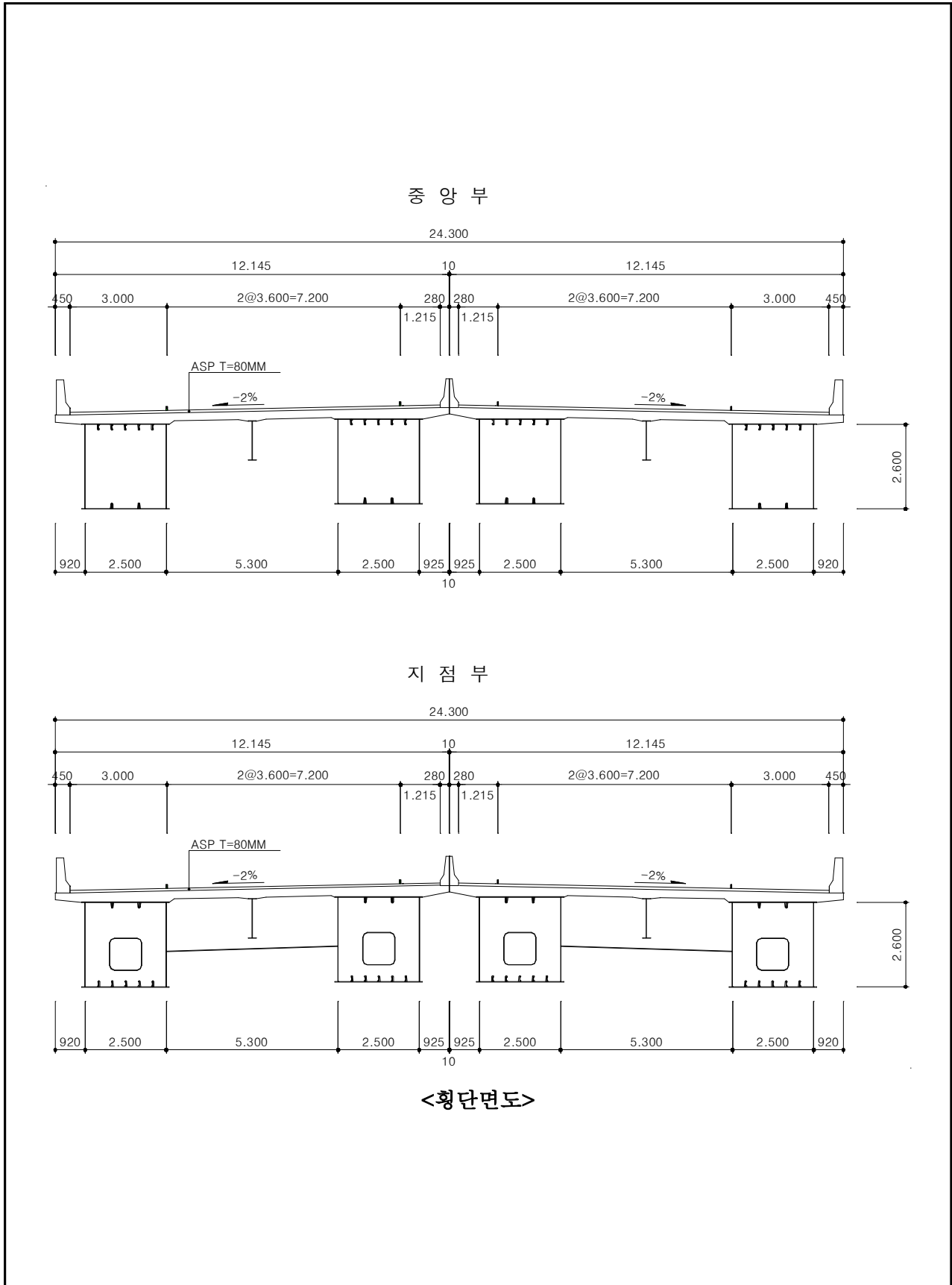
【그림 1.4.2】 남천교 횡단면도
