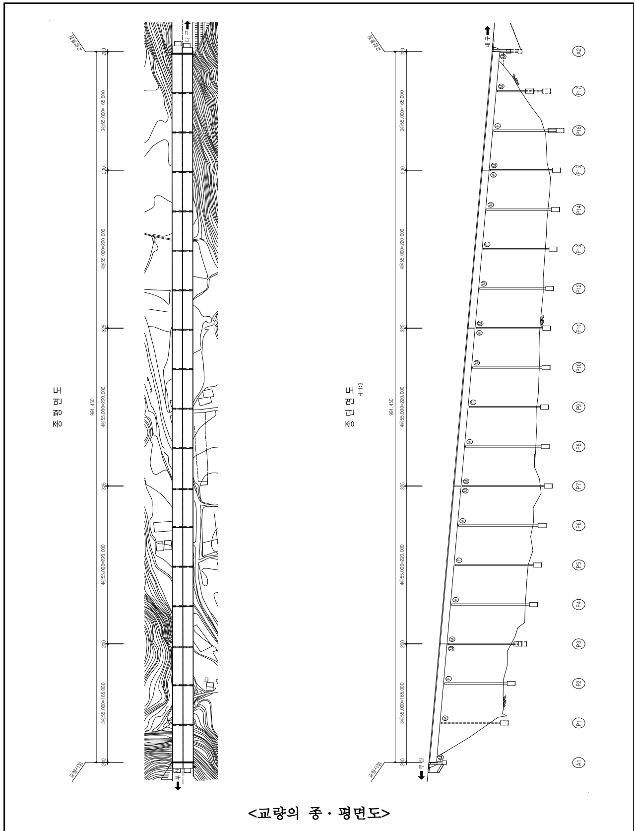
【그림 1.4.1】 남천교 종·평면도
