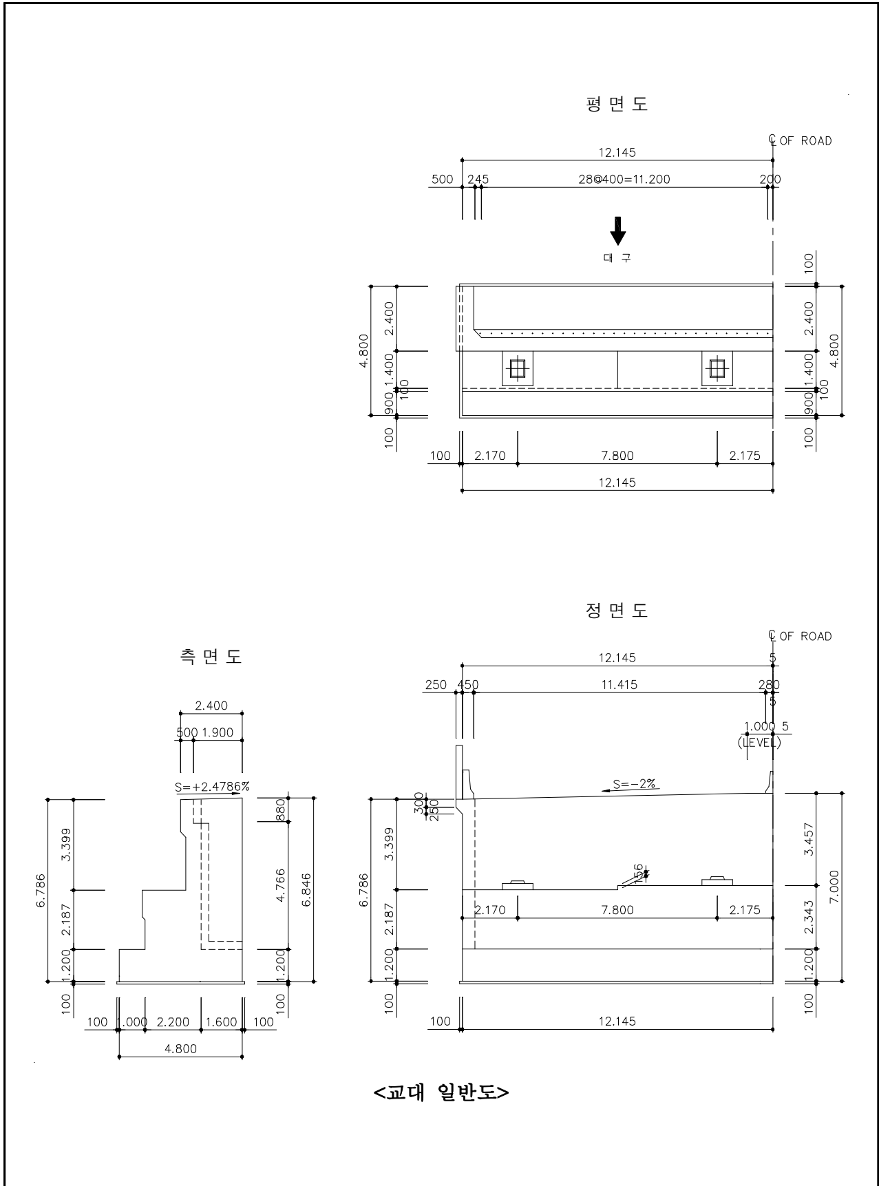
【그림 14.3】 남천교 교대 일반도
